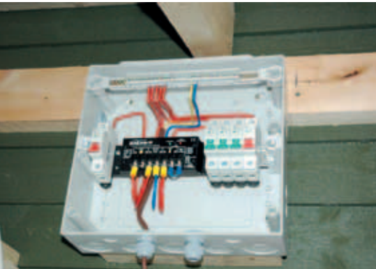
SunSaver-10 avattuna
